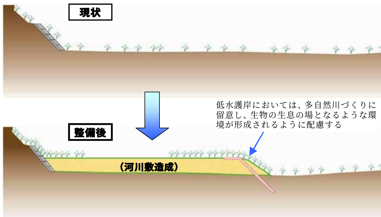
図-4.1.21 堤防の質的強化対策箇所の環境配慮イメージ（その2）
